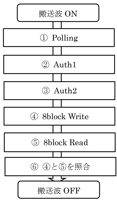
図 6-16 シーケンスソフトウェア
