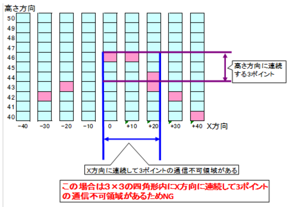
図 6-12 通信不可領域グラフ拡大図（NGパターン②）
