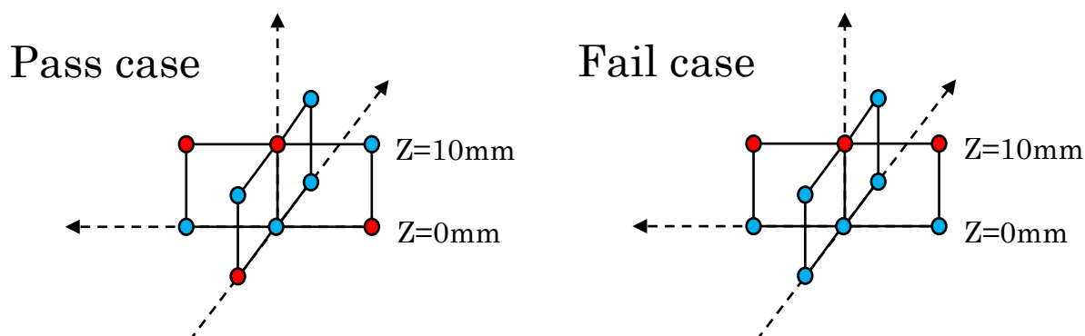
図 6-15 対向外通信測定 合格基準例
