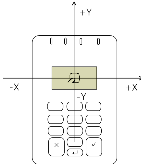
図 6-4 M010 の X 方向、Y 方向
