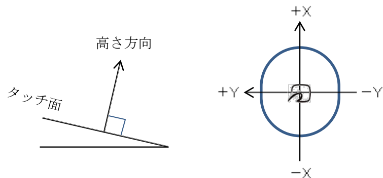
図 6-6 改札機 EG2 (RC-S470C) の X 方向、Y 方向
