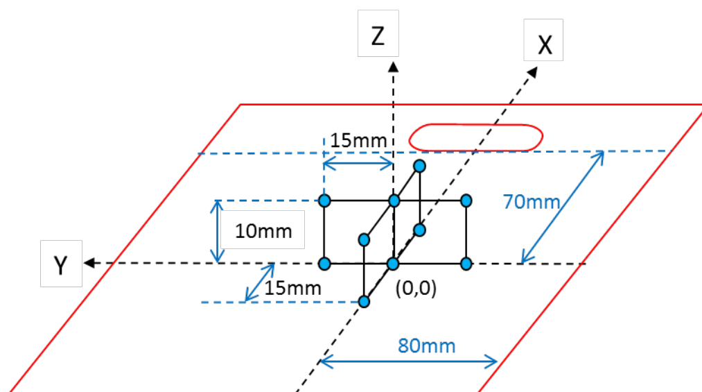
図 6-14 対向外通信測定 測定点
