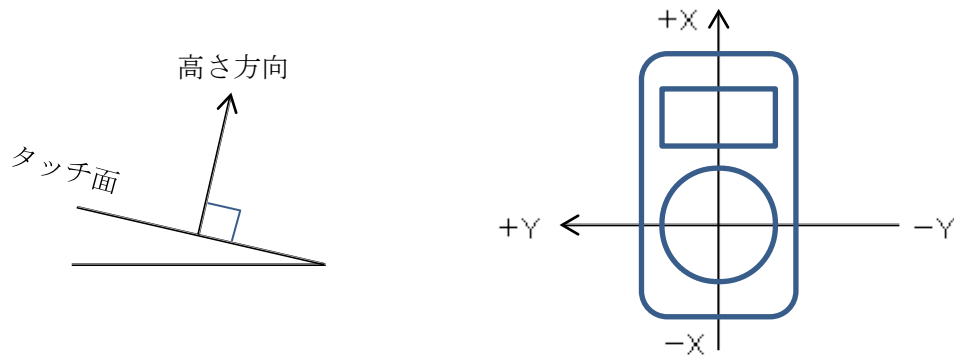
図 6-10 BT2 物販端末ユニット (JT-R591CR-10) の X 方向、Y 方向
