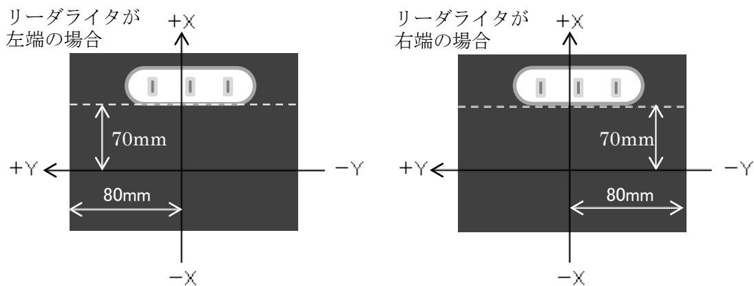
図 6-9 車上リーダーライト（VT-9271A）の X 方向、Y 方向
