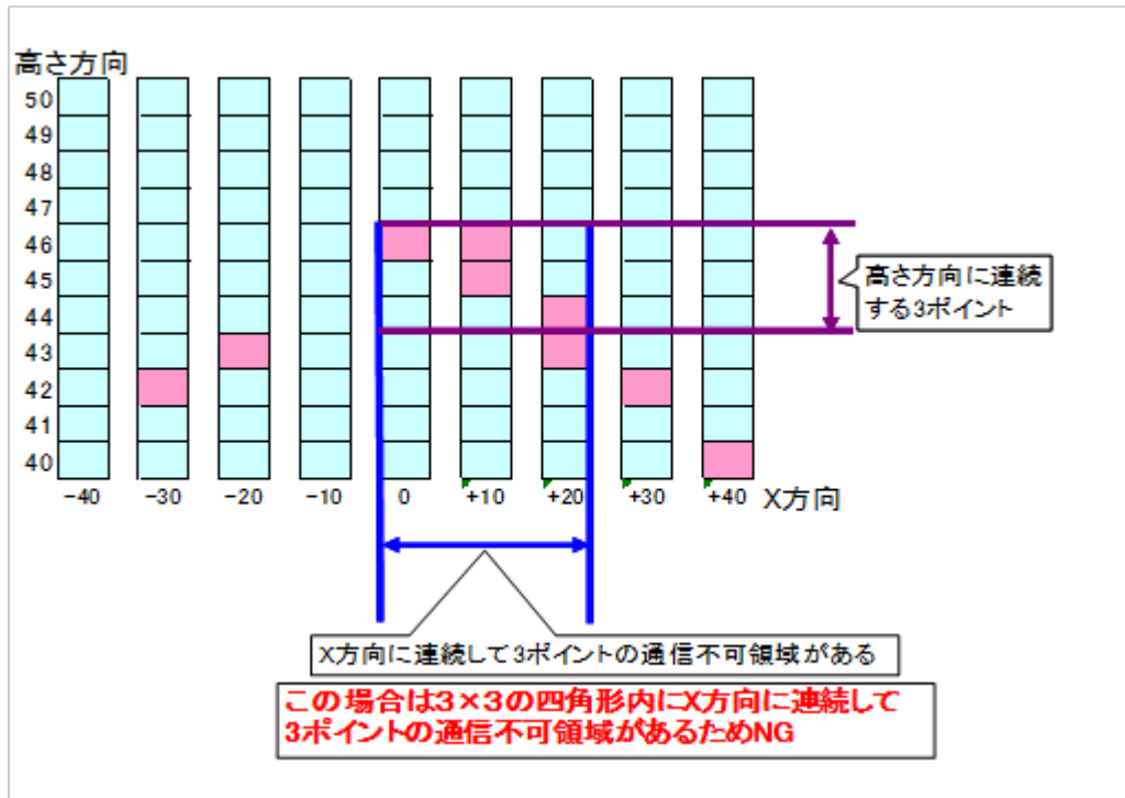
図 6-11 通信不可領域グラフ拡大図（NGパターン①）
