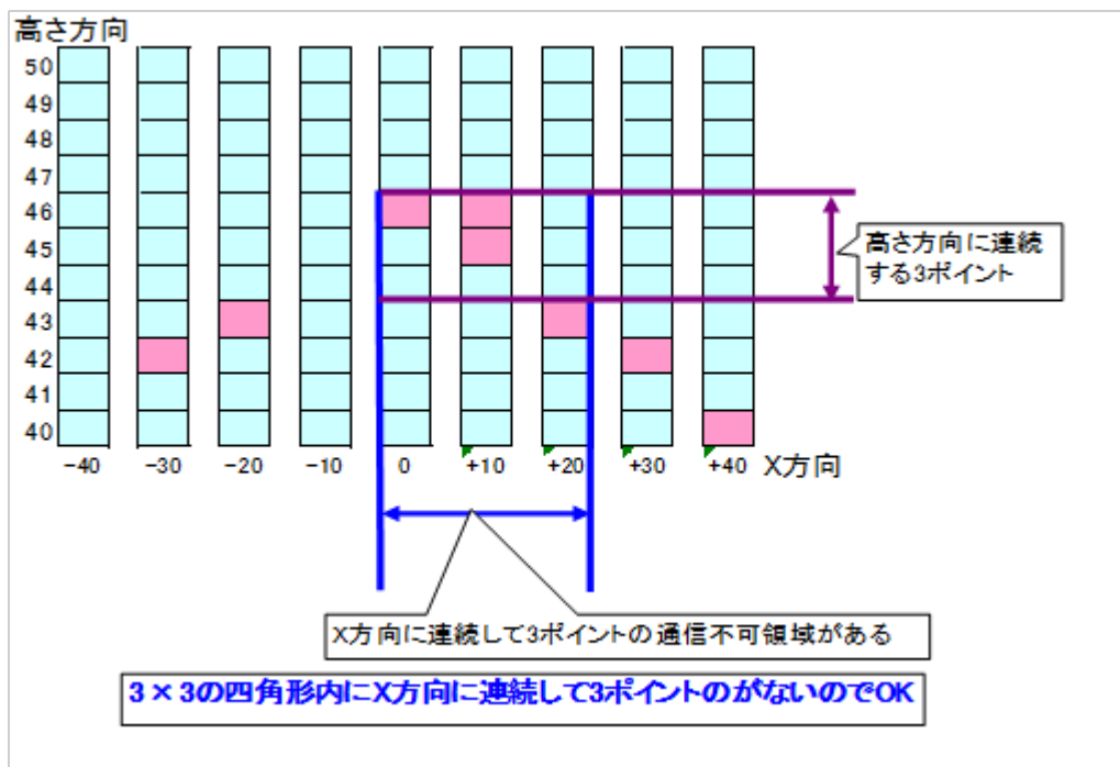
図 6-13 通信不可領域グラフ拡大図（OKパターン）
