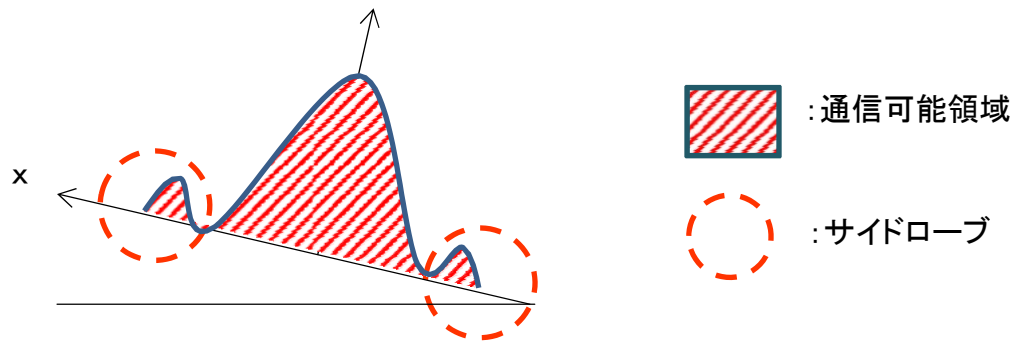
図 8-1 サイドローブ
